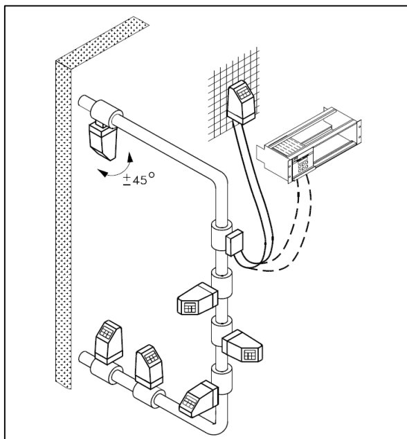
Montaż poziomy
