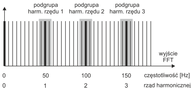
Rys. 39. Wyznaczanie podgrup harmonicznyc (sieć 50 Hz).
