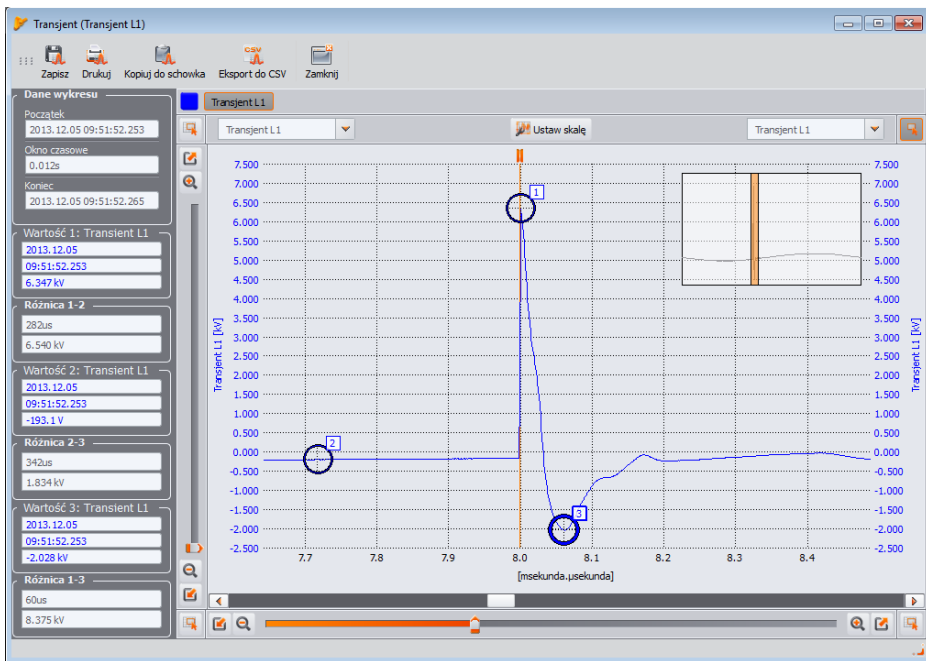
Rys. 54. Przykładowe przebiegię piorunowe.
