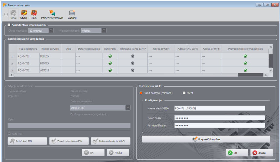
Rys. 31. Ekran konfiguracji punktu dostęowego Wi-Fi.
